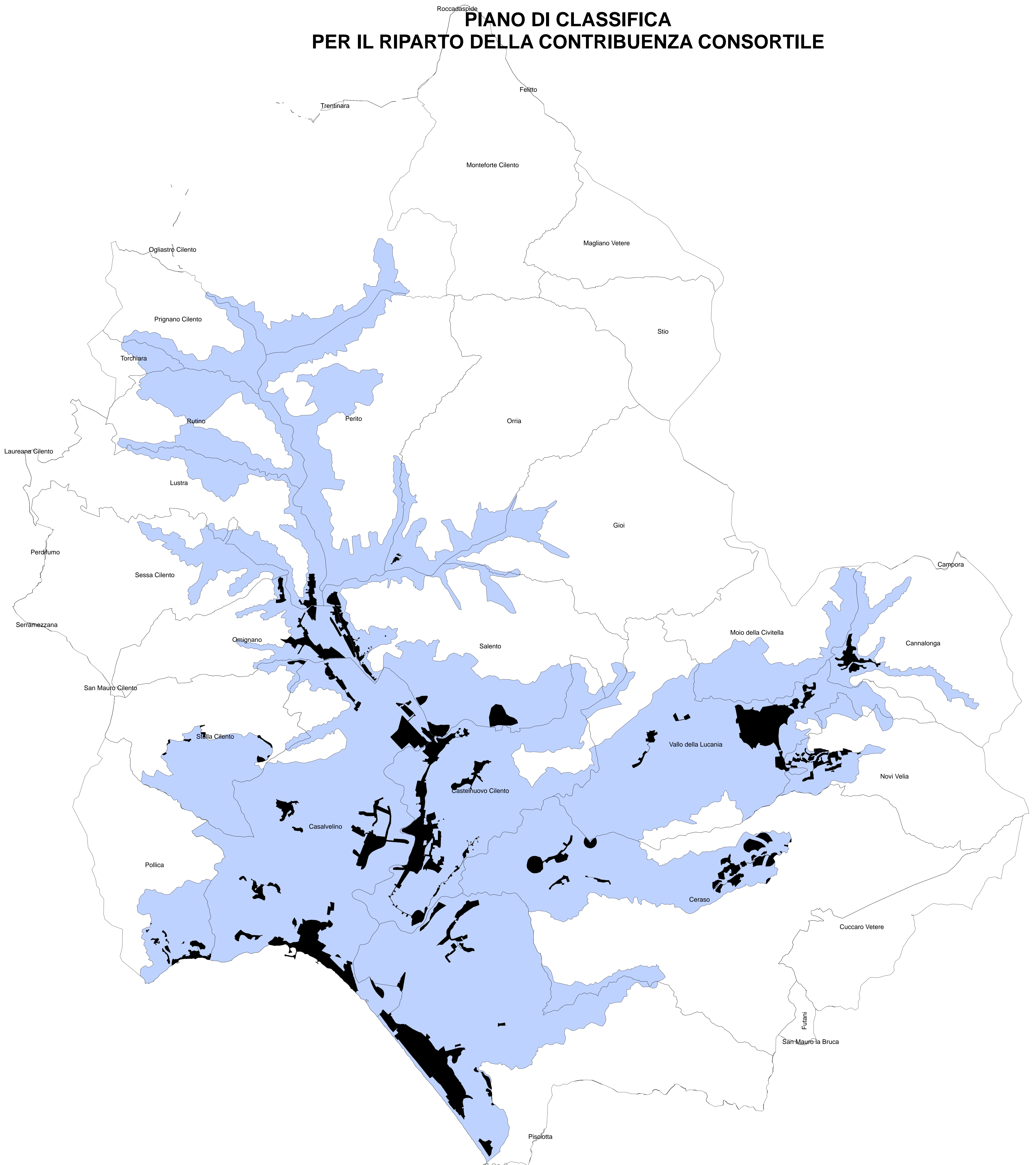
TAV. 11 AREE DI PIANO REGOLATORE A DESTINAZIONE NON AGRICOLA IN CUI SONO PRESENTI UTENZE DEL SERVIZIO DI PUBBLICA FOGNATURA
